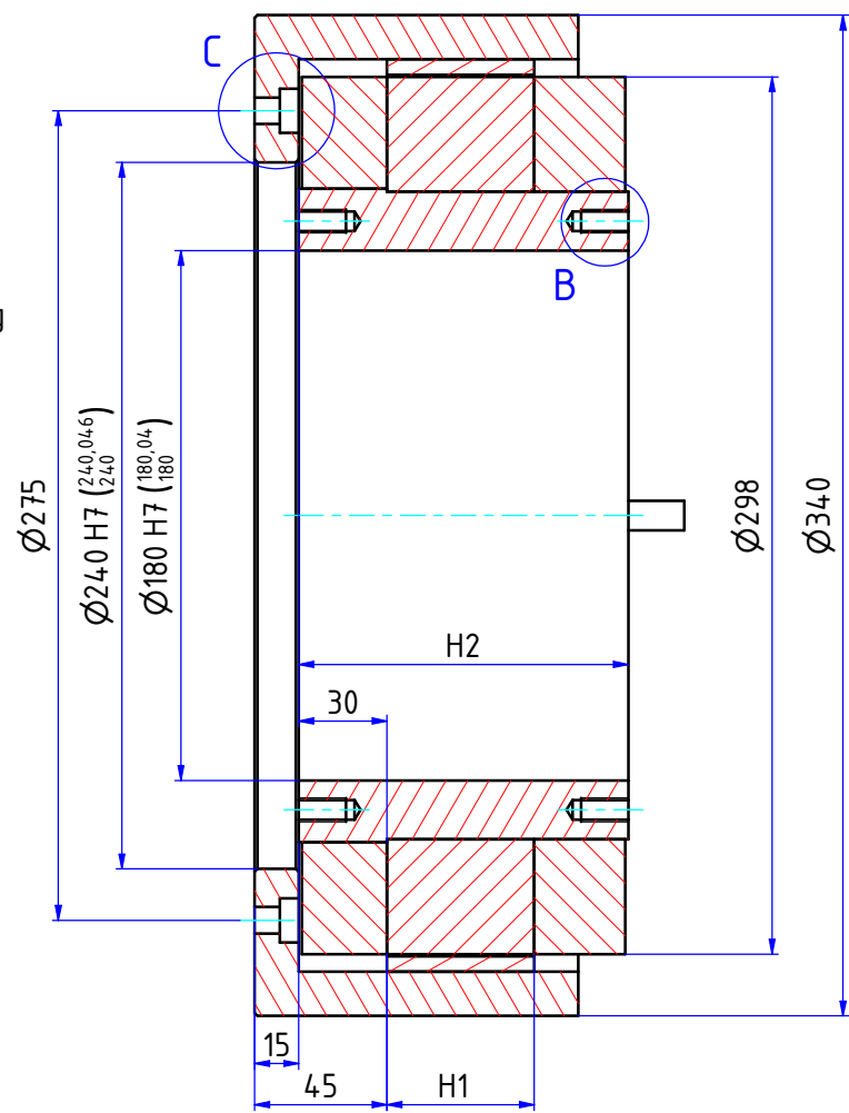
A-A ( 1 : 2 )
