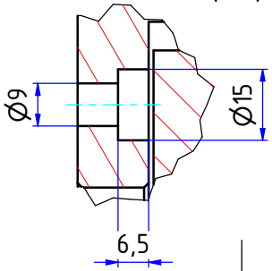
C ( 1 : 1 ) (12x)
