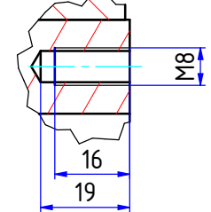
C ( 1 : 1 ) (12x)
